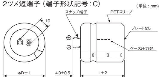
2ツメ短端子 (端子形状記号: C)
