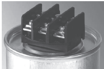
Z3 / S4 端子 (対応ケース径：φ60～136mm)
