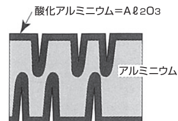
図4 化成箔模型図
