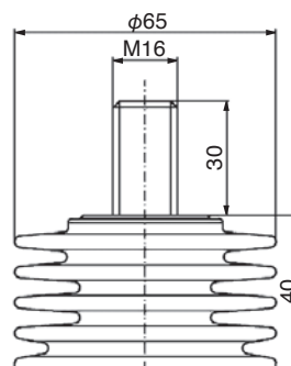
F6 M16×30
