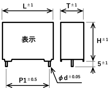
【2-terminals】
