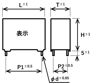
【4-terminals】
